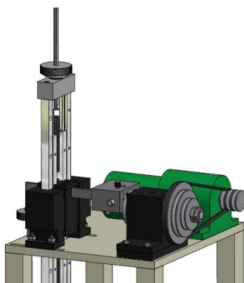
Fig. 2. Tribometer.
